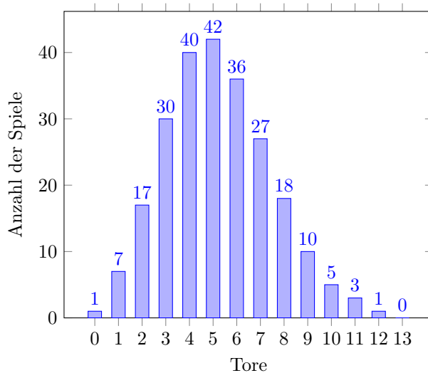
Bild 8: Anzahl der Spiele mit simulierten Toranzahlen: Laut Prof. Metin Tolan lassen sich bei Spielen, bei denen Tore unabhängig voneinander erzielt werden, die Anzahlen der Tore mittels Poisson-Verteilung simulieren. Damit würden sich bei 239 Spielen und 5,25 Toren pro Spiel die in dieser Grafik gezeigten Anzahlen ergeben. Mit unabhängig voneinander ist hier gemeint, dass ein eben erzielt Tor keinen Einfluss auf die Wahrscheinlichkeit des nächsten Torerfolgs hat. Beim Volleyball beispielsweise ist das anders – es geht dort natürlich nicht um einen Torerfolg, sondern einen Punktgewinn –, da ist die Wahrscheinlichkeit dafür, nach einem Punktgewinn den nächsten Punkt zu erzielen, kleiner, weil man ja dann Aufschlag hat und die andere Mannschaft normalerweise die beste erste Chance.
