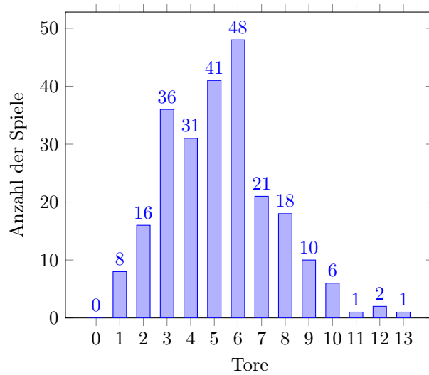
Bild 7: Anzahl der Spiele mit Toranzahlen: Üblicherweise ist hier keine Delle zwischen drei und fünf Toren, sondern die Anzahl der Spiele mit vier Toren liegt dazwischen. Vermutlich sind 239 Spiele ein bisschen wenig für eine verlässlichere Statistik – siehe Bild 8 auf Seite 9 für eine weitere Anmerkung.
